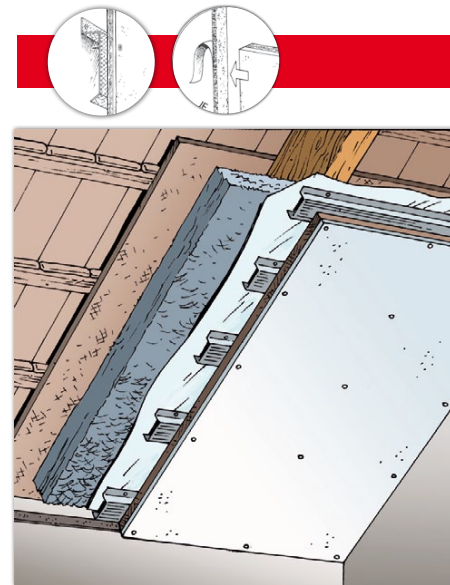
Extension essai CEDIA 06/4861 Sous toiture : R_w(C;Ctr) = 52(-2; -8) dB
