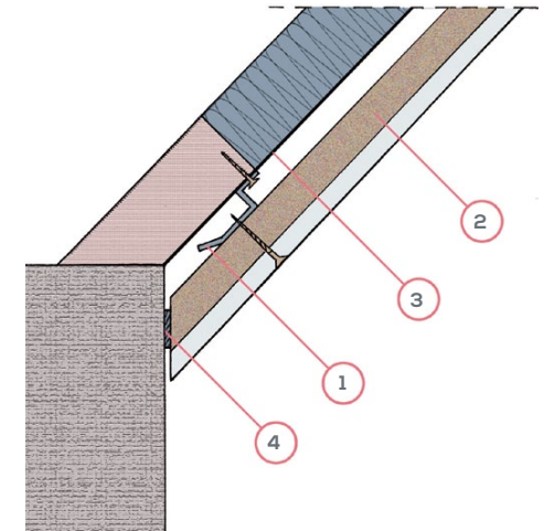
Extension essai CEDIA 06/4861 Sous toiture : R_w(C;Ctr) = 52(-2; -8) dB
