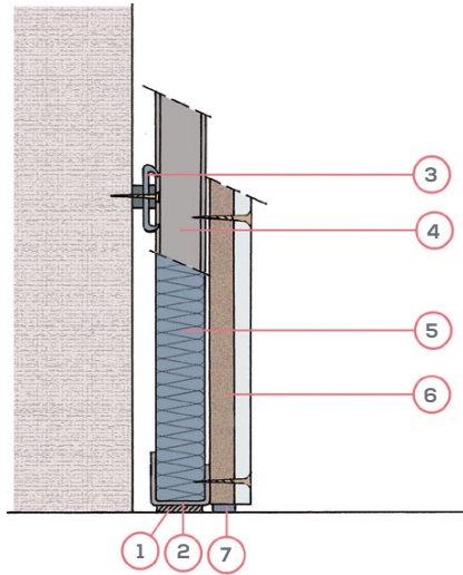
Extension essai CEDIA 08/5343 Cloison de référence : R_w(C;Ctr) = 32(-0;+2) dB Cloison doublée sur antivibratoire : R_w(C;Ctr) = 56(-2;+7) dB
