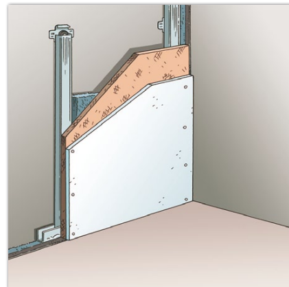
La Fixation Antivibratoire Réf. FA 60
