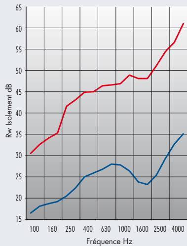
Essai CEDIA CEDIA 2010/56 58 Plancher bois : R_w(C;Ctr) = 26(-1; -2) dB Plancher et plafond : R_w(C;Ctr) = 48(-2; -5) dB
