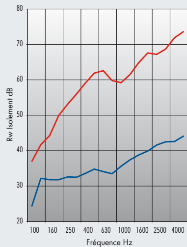
Extension essai CEDIA 08/5343 Cloison de référence : R_w(C;Ctr) = 32(-0;+2) dB Cloison doublée sur antivibratoire : R_w(C;Ctr) = 56(-2;+7) dB
