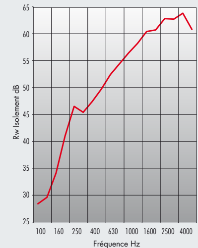
Extension essai CEDIA 06/4861 Sous toiture : R_w(C;Ctr) = 52(-2; -8) dB
