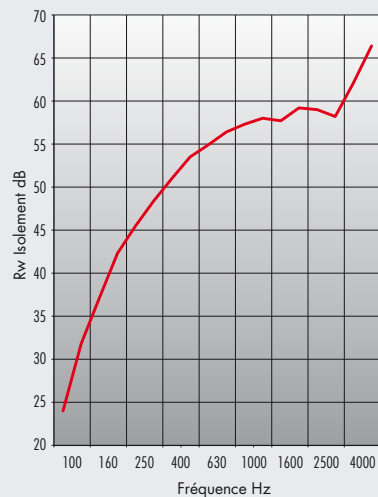
Essai CEDIA 2011/5912 - Rw(C ;Ctr) = 54 (-4 ; -11) dB
